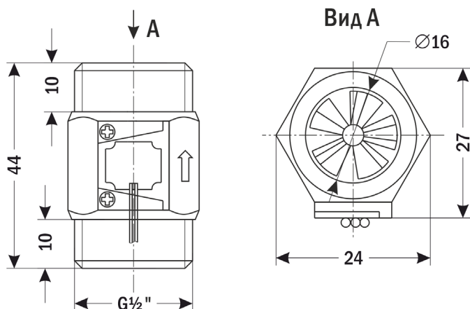
Рис. 2 – Размеры прибора
